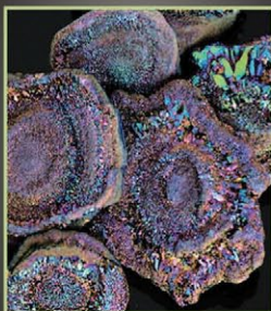
GALAXY DRUZY
